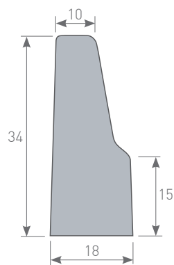
Élément droit : Long. 1 m - Poids : 108 kg
